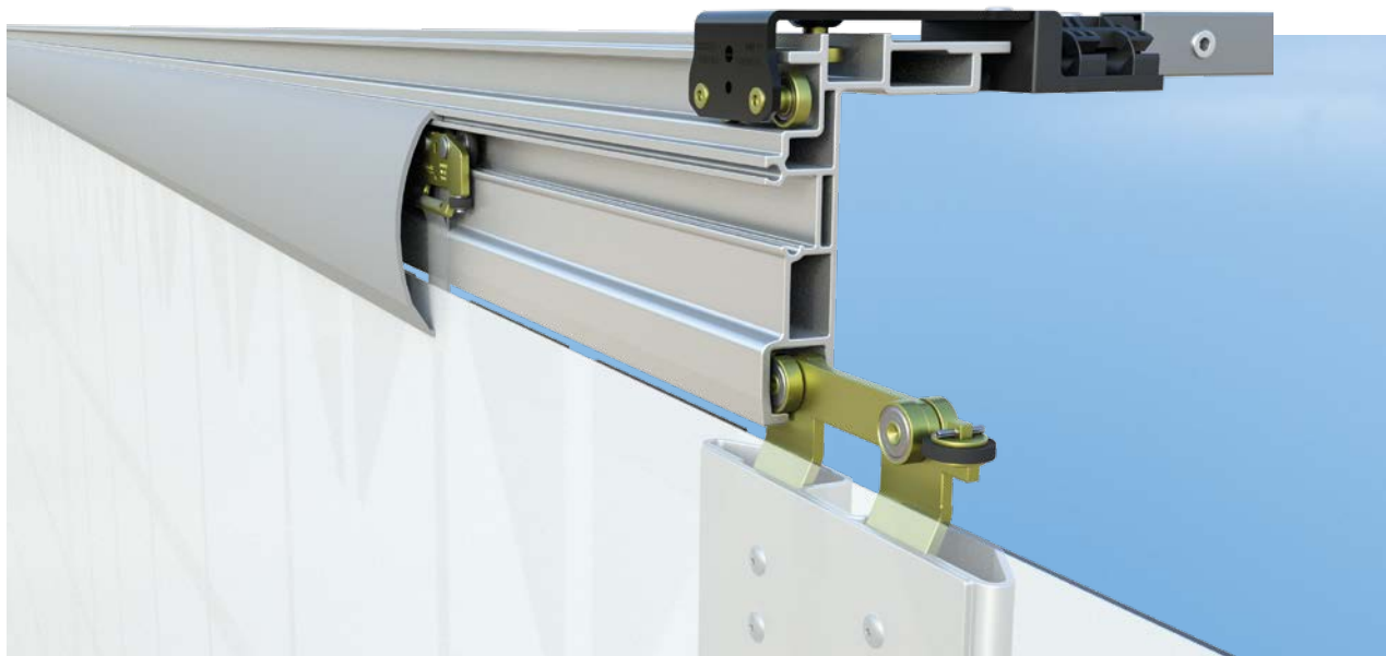
Systemaufbau System structure
