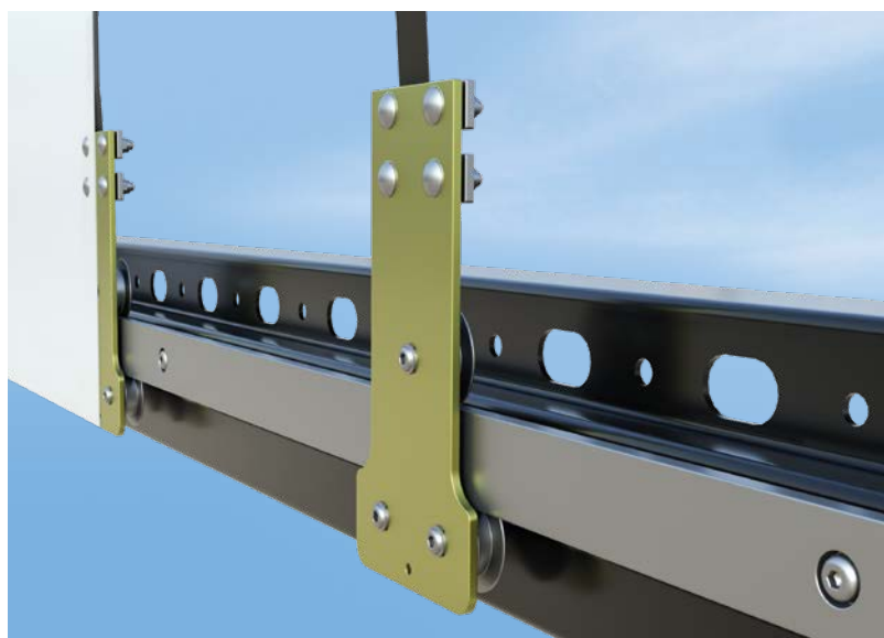
Führung Laufrollen unten, Außenseite Guidance for rollers bottom, outside
