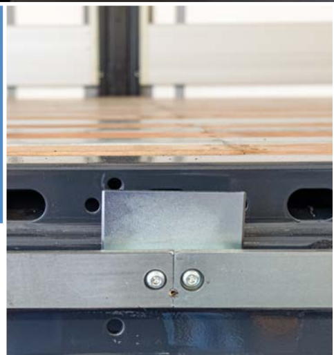
Geteilte Schienen und Momentenabstützung Split rails and moment support
