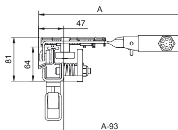
Profil MEGALINER Profile MEGALINER
