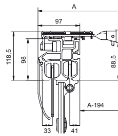
Profil MULTILINER Mix Profile MULTILINER Mix
