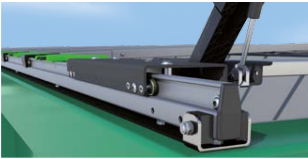
komplett auf E-Wagen verschraubt fully rigged to E-wagon
