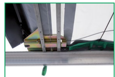
Hinteres Verdeckende mit Edscha TS-Portalbalken, Seilanbindung und Verriegelung Rear end of roof with Edscha TS gantry beam, cable connection and lock
