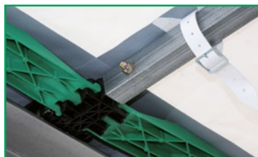
Drehpunkt mit Clipverbindung Pivot point with clip connection
