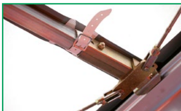
Rollenwagen mit Seilanbindung und Planenbefestigung Glider with cable connection and tarpaulin attachment
