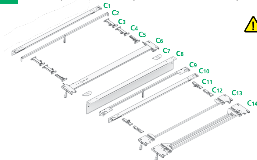
Endlaufwagen Front für beidseitige Verschiebbarkeit · End Carriage front for bidirectional moving
