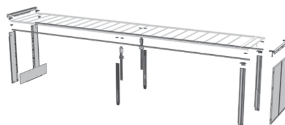
Algunos de los componentes de la superestructura
