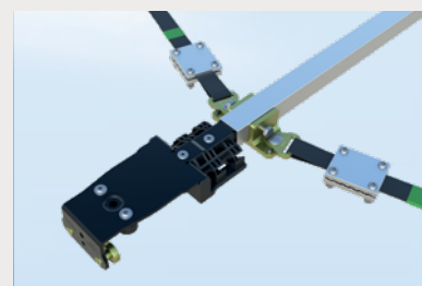
Cinchas ajustables EN 12642 XL
