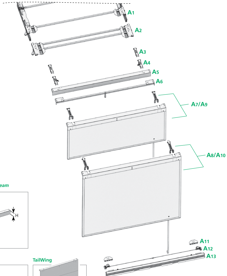
Montagesatz hinten Assembly kit rear
